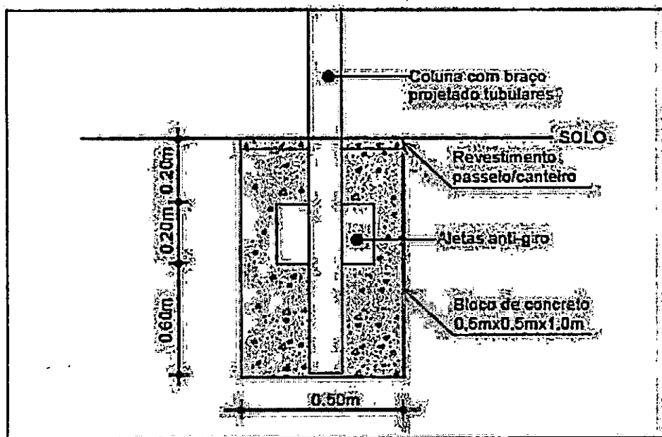
Figura 03 – Fixação do suporte TIPO III no solo
