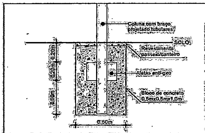
Figura 03 – Fixação do suporte TIPO III no solo
