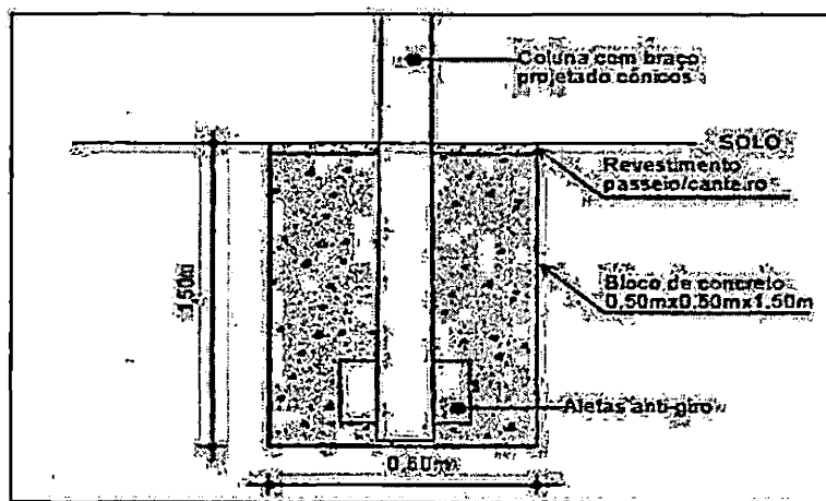
Figura 02 – Fixação do suporte TIPO II no solo
