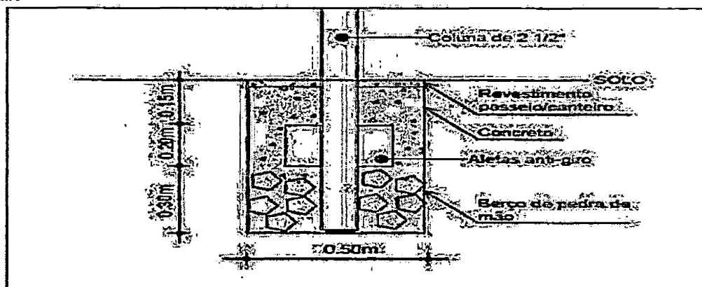
Figura 01 – Fixação do suporte TIPO I no solo
