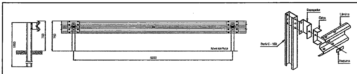
Figura 2. Modelo da defesa metálica semi-maleável simples.
