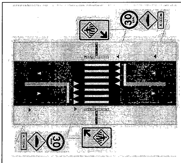
Figura 1. Modelo da Faixa Elevada de Pedestres
